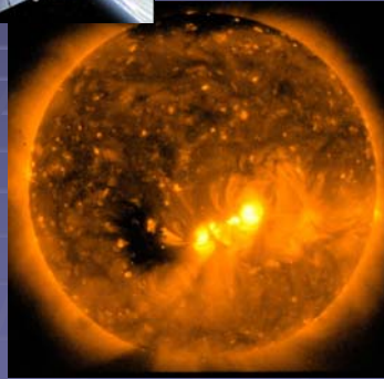
ひのでがX線でみた太陽
