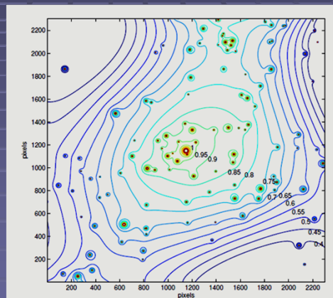
重力レンズ法による銀河団 MACS J1149の質量分布
