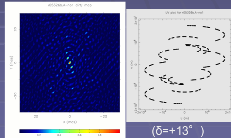
通常のVERA(4局6基線)のUVとビーム
