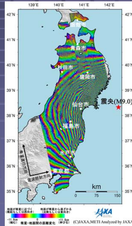
3月11日の地震による地殻変動
