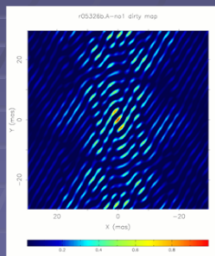
VERAの水沢一入来基線のUVとビーム
