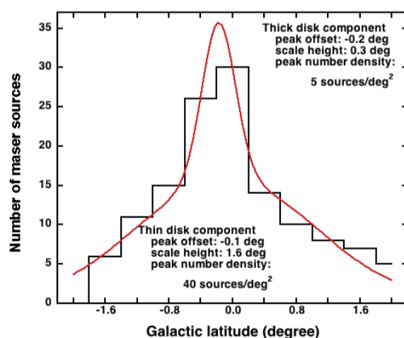
図7 1612 MHz OH メーザー源分布に見られる銀緯方向に対する依存性。2つのガウス型度数分布の重ね合わせ。銀河中央面のデータ群は大質量星形成領域に付随するものに相当し、それ以外のウィング成分は OH/IR 星起源だと考えられる (他データによる同定と比較が必要)。
