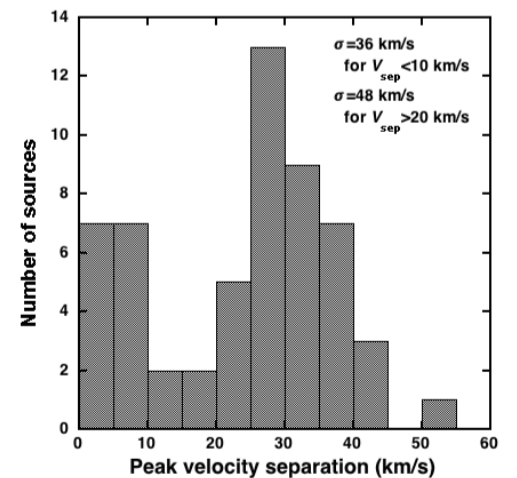
図8 ダブルピークプロファイルを持つと判定された 1612 MHz OH メーザー源のピーク間速度差 (= 膨張速度 × 2) 分布。膨張速度が2分化しているのは、大質量星形成領域と OH/IR 星のサンプル群に分かれているからだと考えられる。
