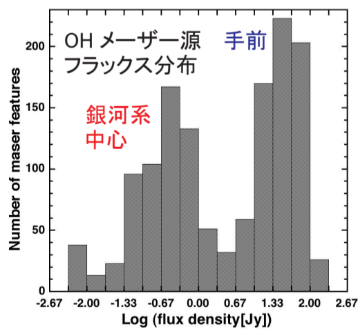
図6 GASKAP 観測検討時のシミュレーションから得られた銀河系中心方向 (4° . 2 四方) で検出される 1612 MHz OH メーザーのフラックス密度度数分布 (Dickey et al. 2013)。手前のメーザー源については既知のメーザー源に対する度数分布である。
